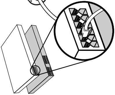
オプションB: パワーオーバーイーサネット (PoE)
